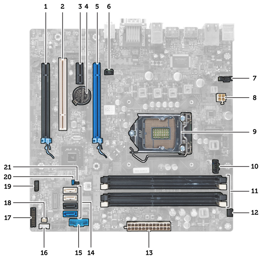
図 1. システム基板のコンポーネント
